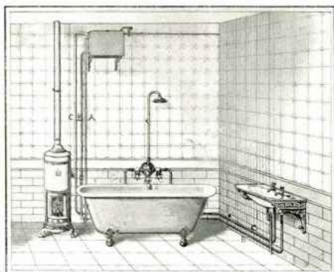
A. Tuyau de trop plein | B. Eau froide. | C. Eau chaude.
