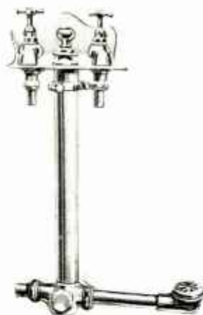
N° 864. Vidage "américain" avec plaque équerre, 2 robinets d'alimentation, siphon orientable.
