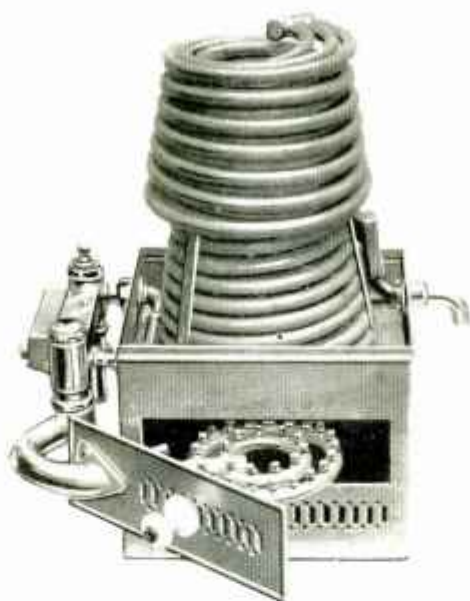
VUE INTERIEURE DES DISTRIBUTEUR "HÉBÉ" SANS SES ENVELOPPES.
